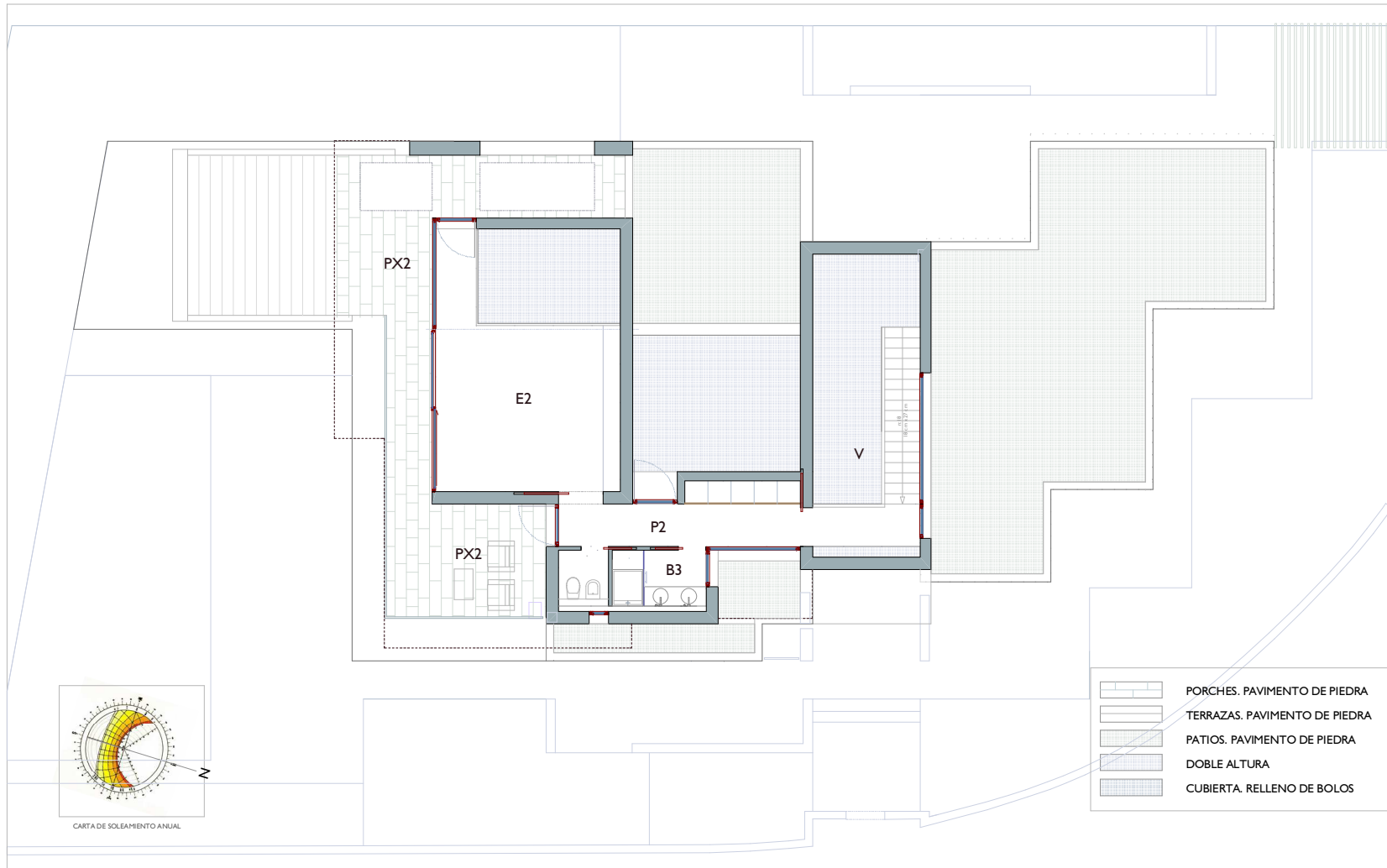
SUPERFICIES PLANTA DE PISO I
