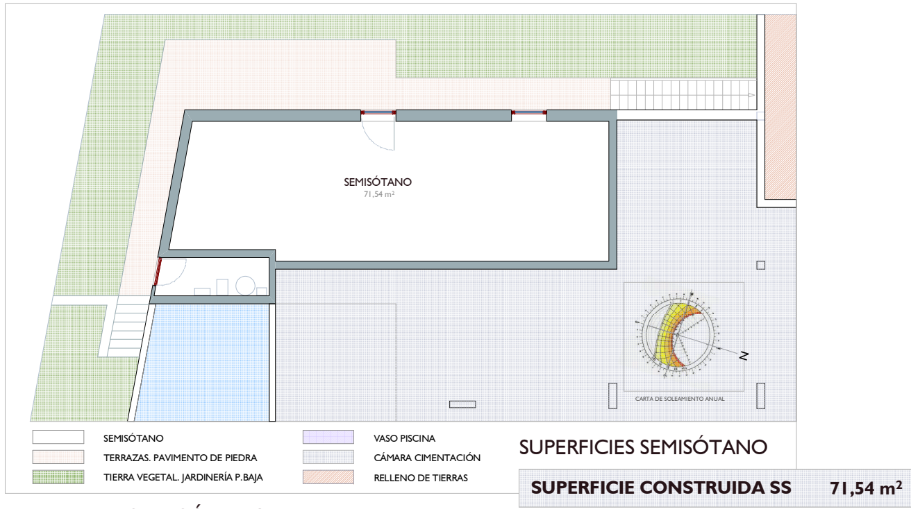
PLANTA SEMISÓTANO
